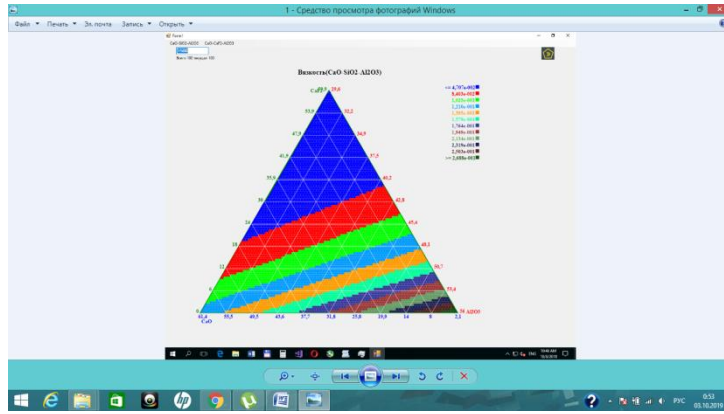
Рисунок 1 – Диаграмма вязкости тройной системы \text{CaO-Al}_2\text{O}_3\text{-SiO}_2 при 1500^\circ\text{C}
