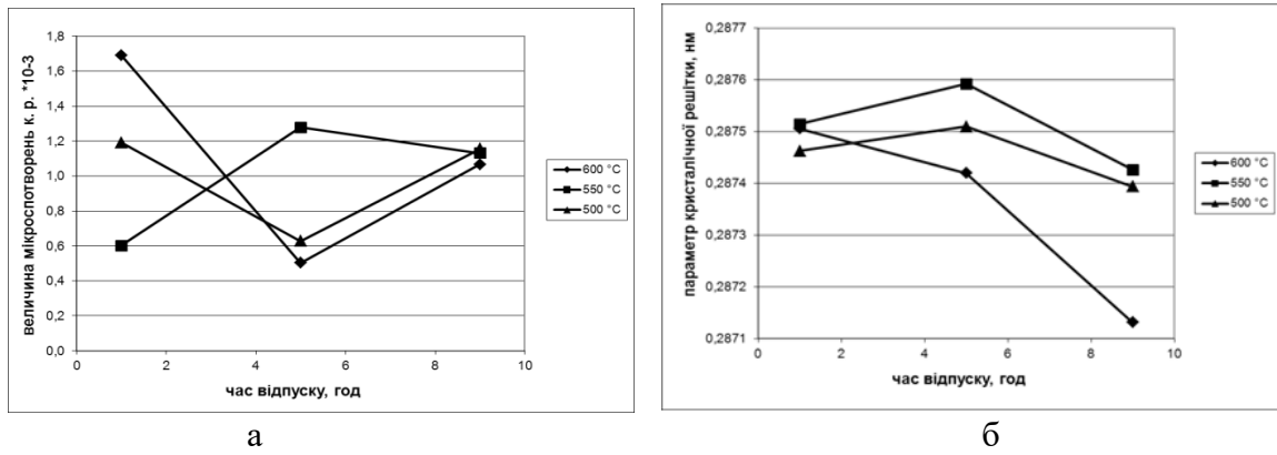
Рис. 2. Зміна величини мікростворень (а) і параметра кристалічної решітки (б) при відпусканні сталі 25Х2М1Ф
